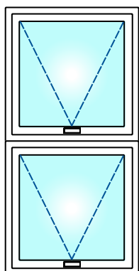
JANELA MAXIM-AR 2 FOLHAS VERTICAL
